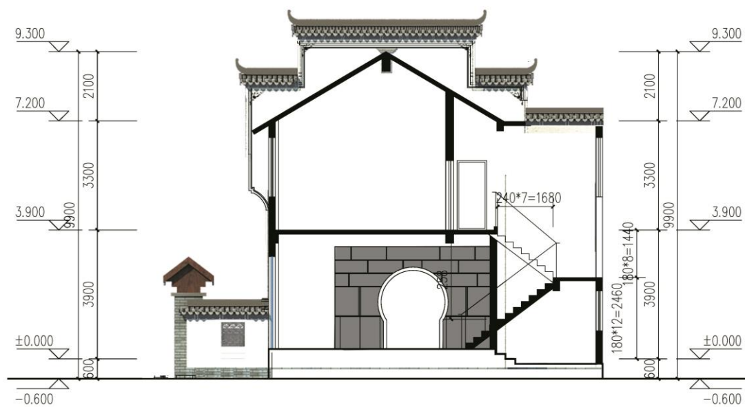
剖面图
